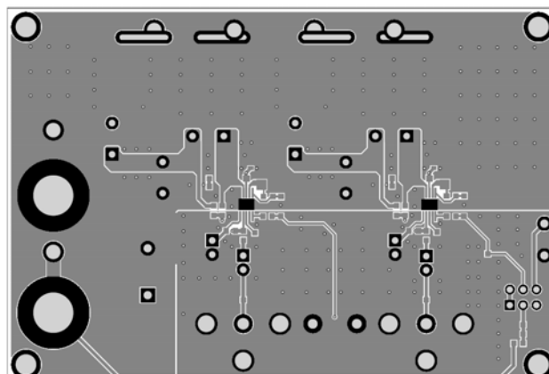
Figure 2—Top Layer
