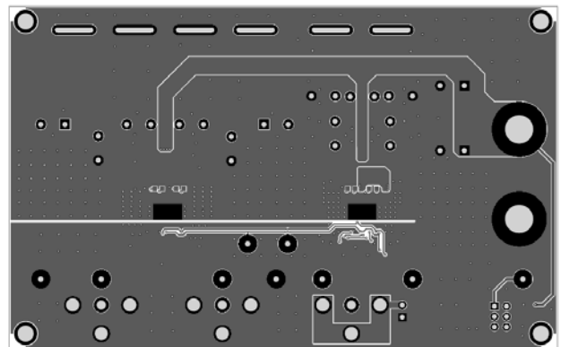
Figure 4—Bottom Layer
