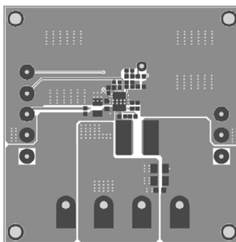
Figure 2—Top Layer
