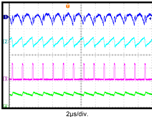
Input/Output Ripple
