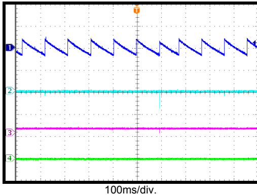
Input/Output Ripple
