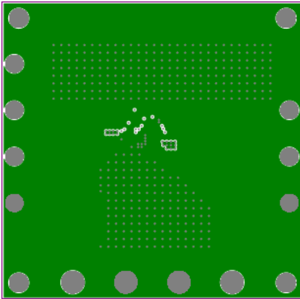
Figure4: Inner1 Layer
