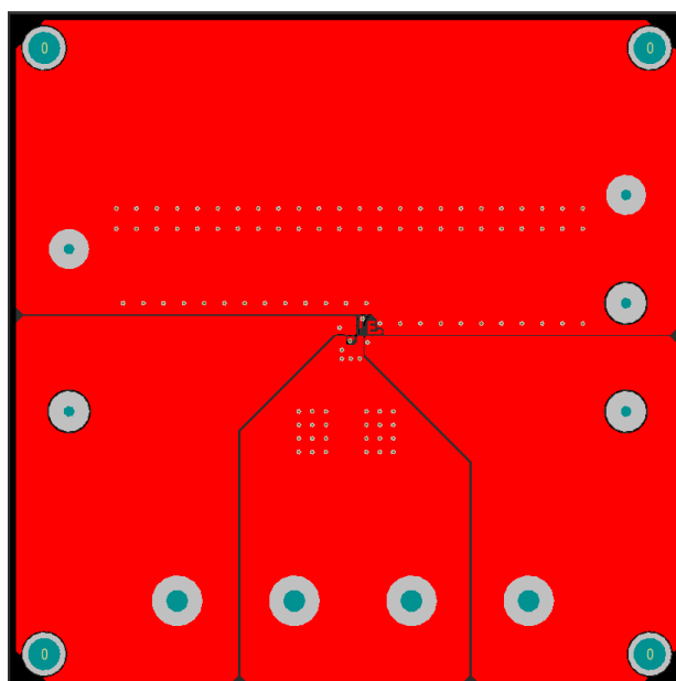
Figure 3—Top Layer
