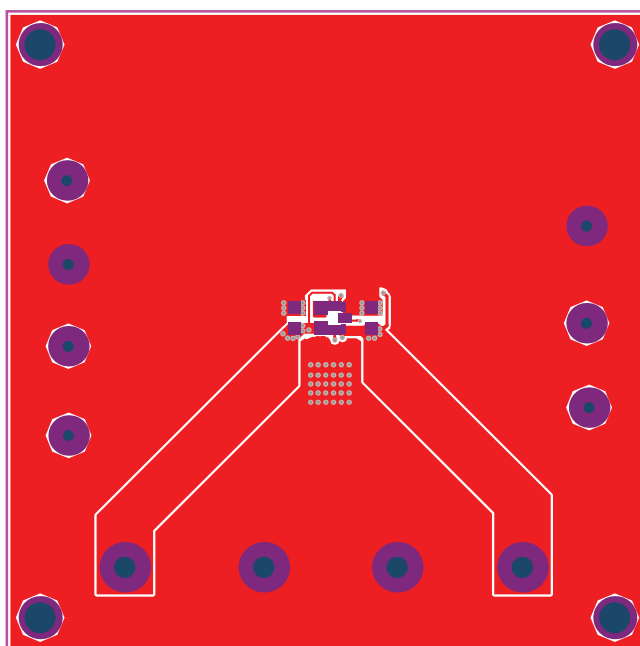
Figure 4—Top Layer
