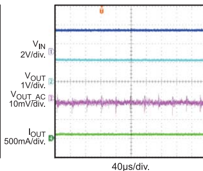
Enable Off
