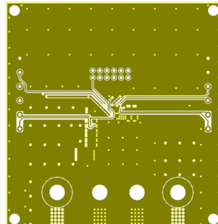
Figure 4— Inner Layer 2
