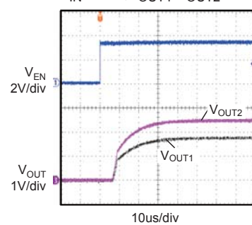
EN Start Up Waveform
