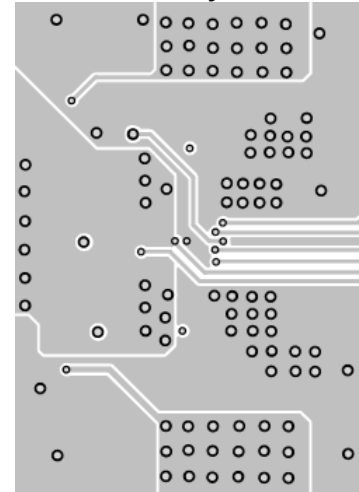
Inner Layer 2
