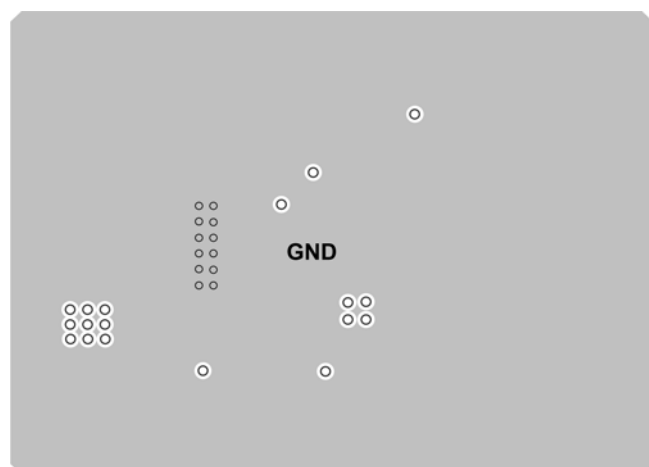
Inner Layer2
