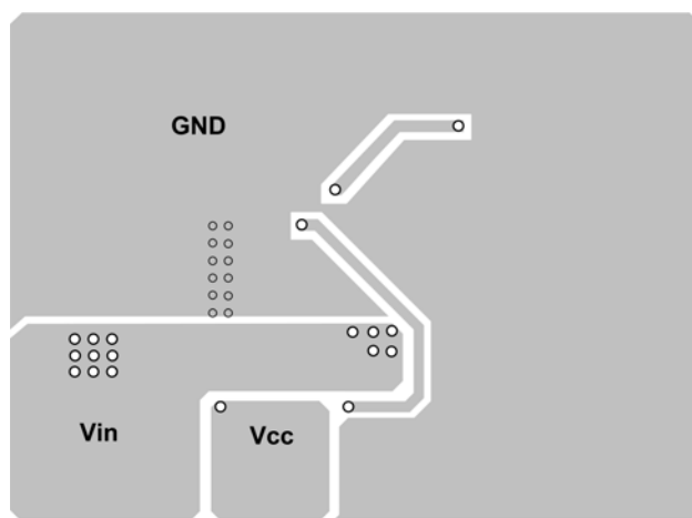
Bottom Layer
