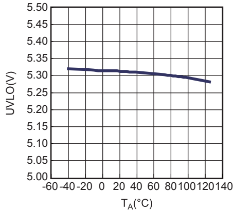
VIN UVLO
