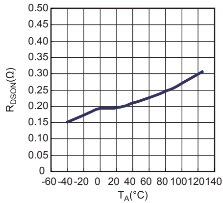
RDSON
