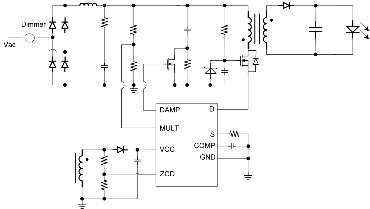
SOIC8
