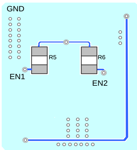
Bottom Layer
