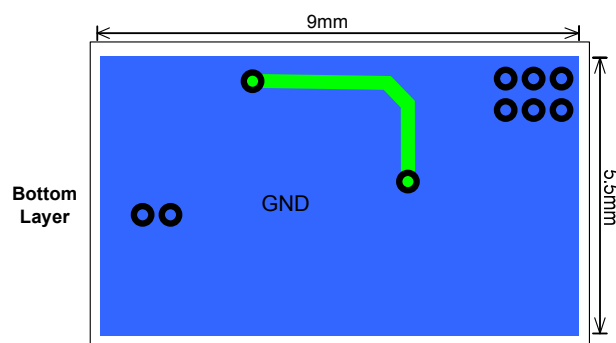
Figure 4— Bottom Layer
