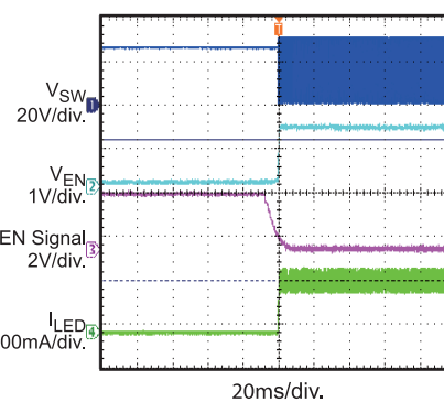
Ven Startup
