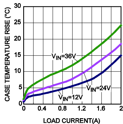
Thermal Rise
