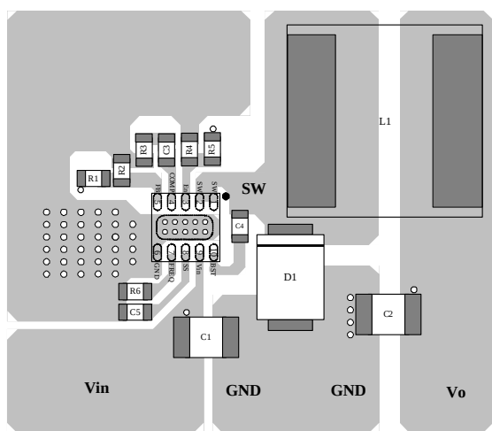
TOP Layer
