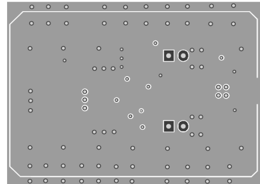
Inner Layer 1
