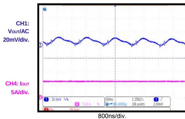
V_{OUT} Ripple
