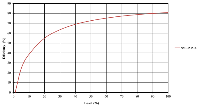
15V Inputs
