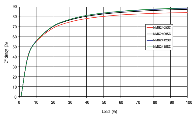
24V Input
