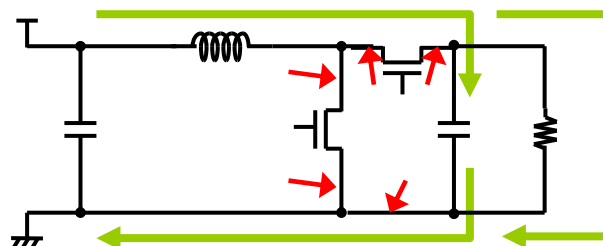
PMOSFET-ON
