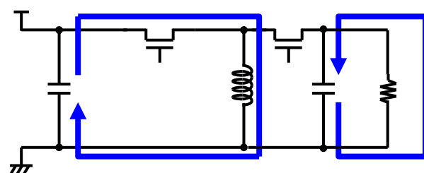
PMOSFET-ON
