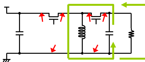
NMOSFET-ON
