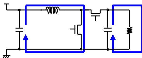
NMOSFET-ON
