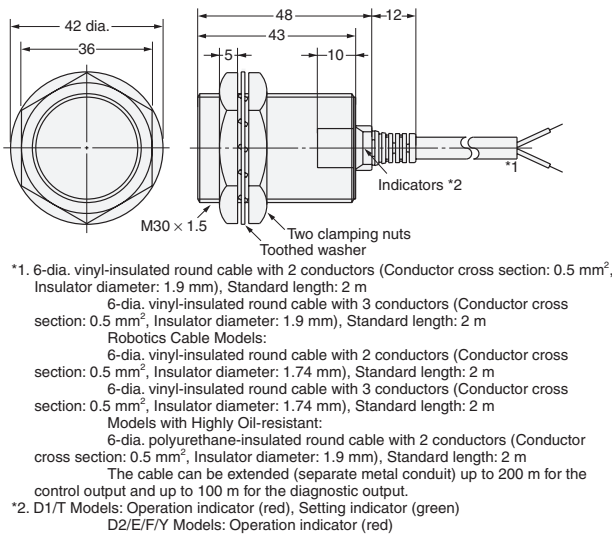
Diagram 12 E2E-X10D□/E2E-X10E□/F□ E2E-X10Y□/E2E-X10T1
