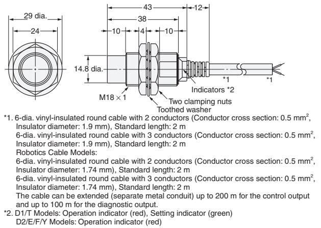
Diagram 11 E2E-X14MD□/E2E-X10ME□/F□ E2E-X10MY□
