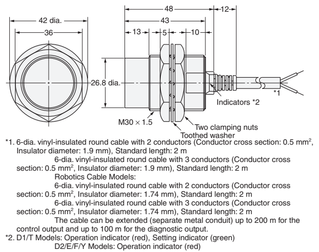
Diagram 13 E2E-X20MD□/E2E-X18ME□/F□ E2E-X18MY□
