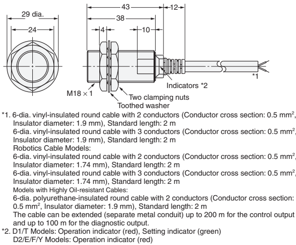
Diagram 12 E2E-X10D□/E2E-X10E□/F□ E2E-X10Y□/E2E-X10T1
