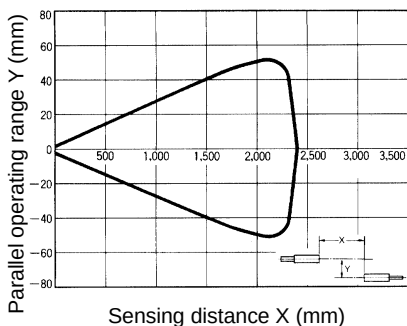
E32-T22S with E3X-NH amplifier
