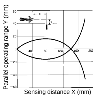
E32-D11R with E3X-NH amplifier
