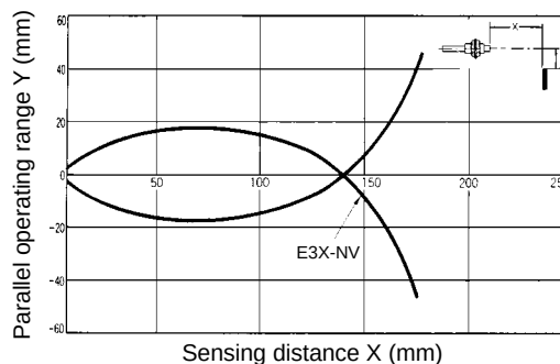
E32-DC200 with E3X-NV amplifier
