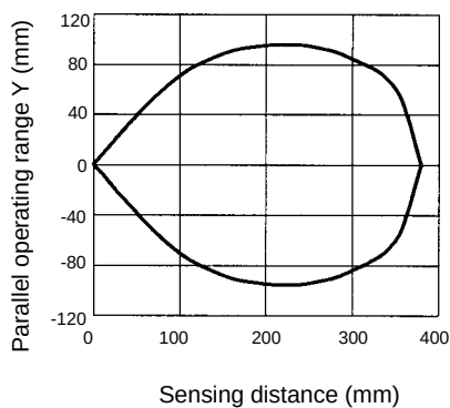
E32-UTBT1-6F with E3JU-X amplifier
