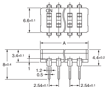
Flat Actuator
