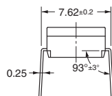
Flat Actuator
