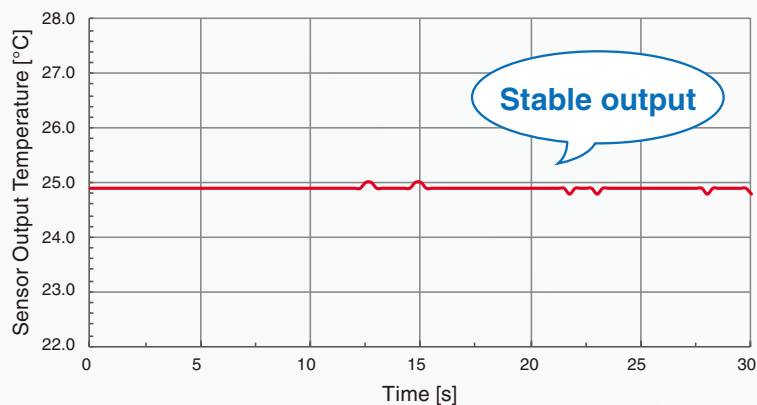
OMRON D6T-1A-01
