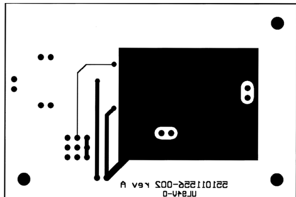
Bottom Layer
