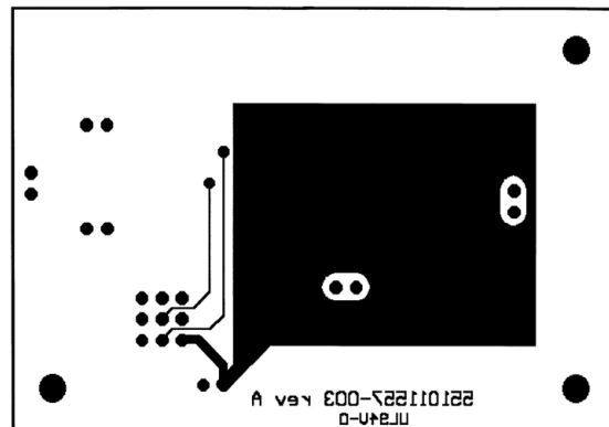
Bottom Layer
