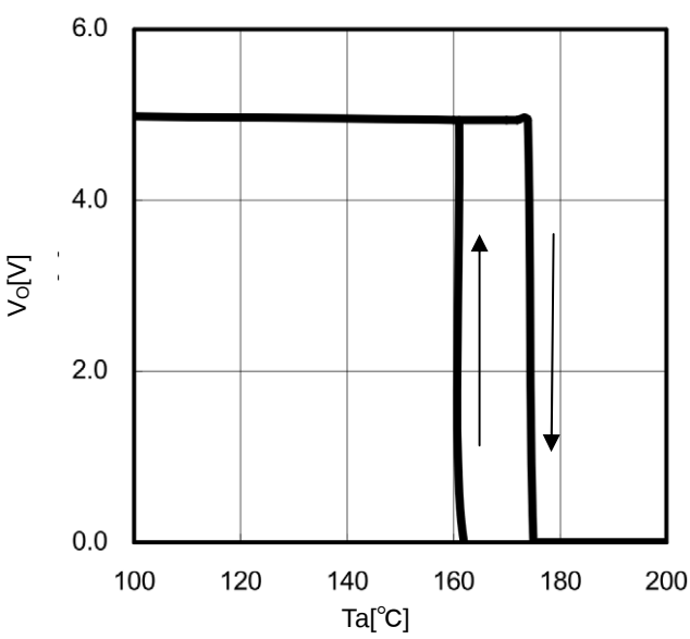
Figure 28. TSD (Io=0mA)
