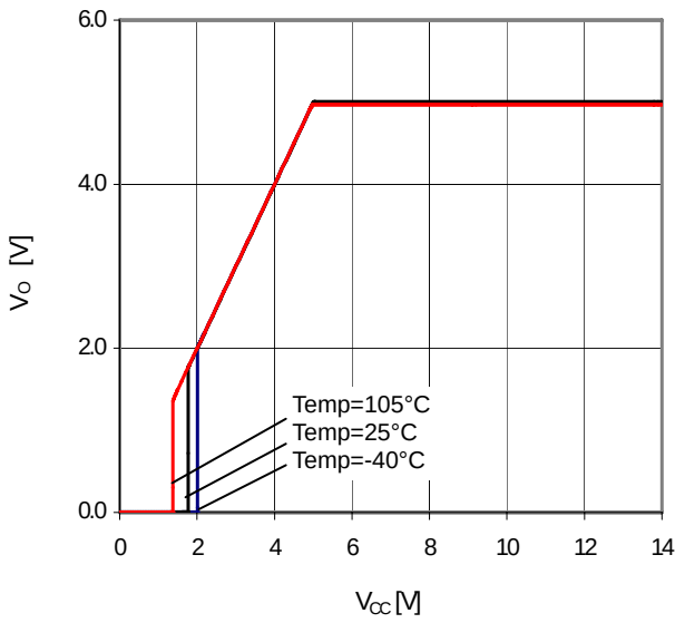
Figure 27. V_{CC}-V_O ( I_O=0\text{mA} )
