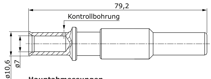
Hauptabmessungen Kontaktstift
